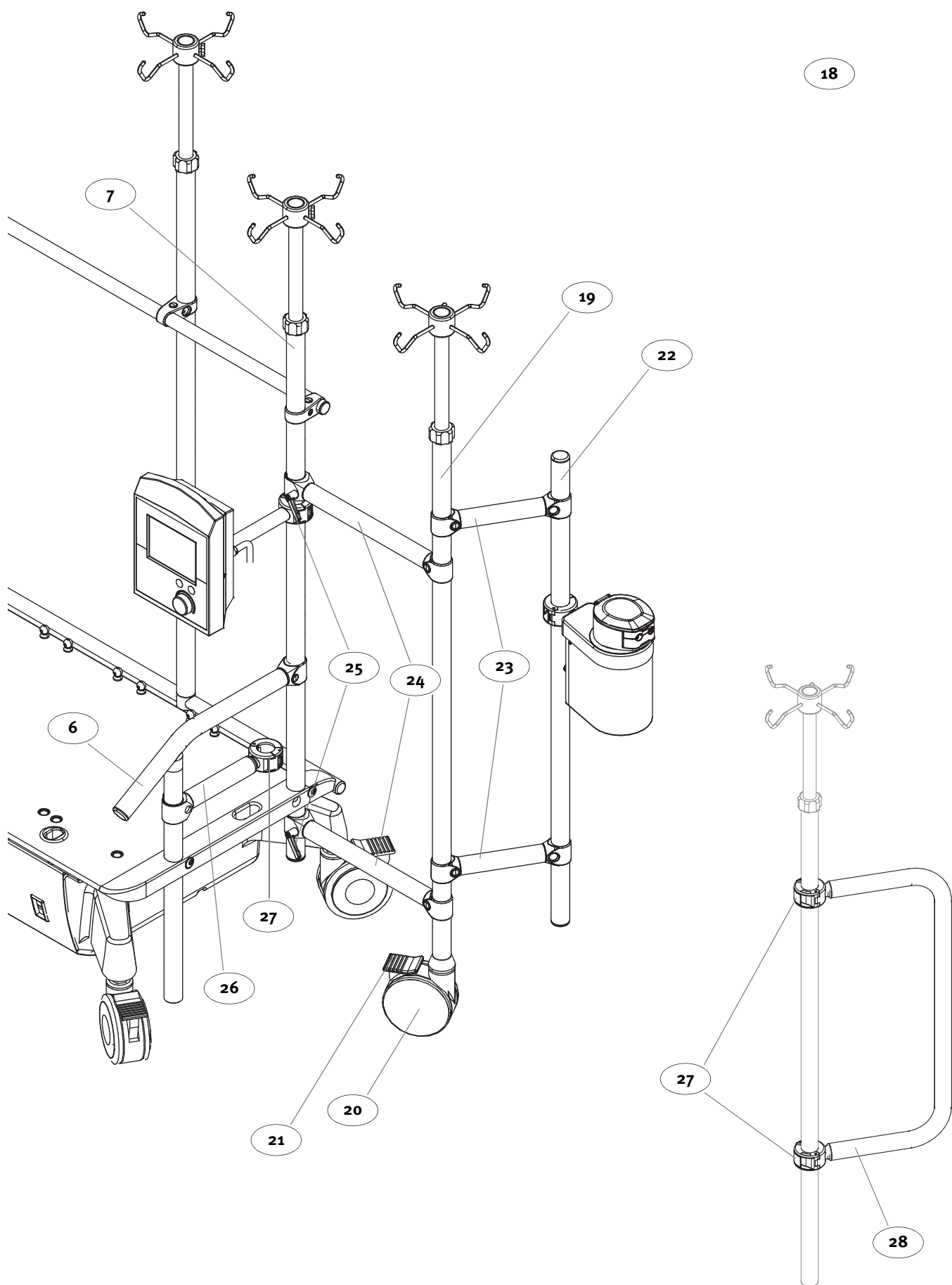
図 2: S5 拡張マストシステム
